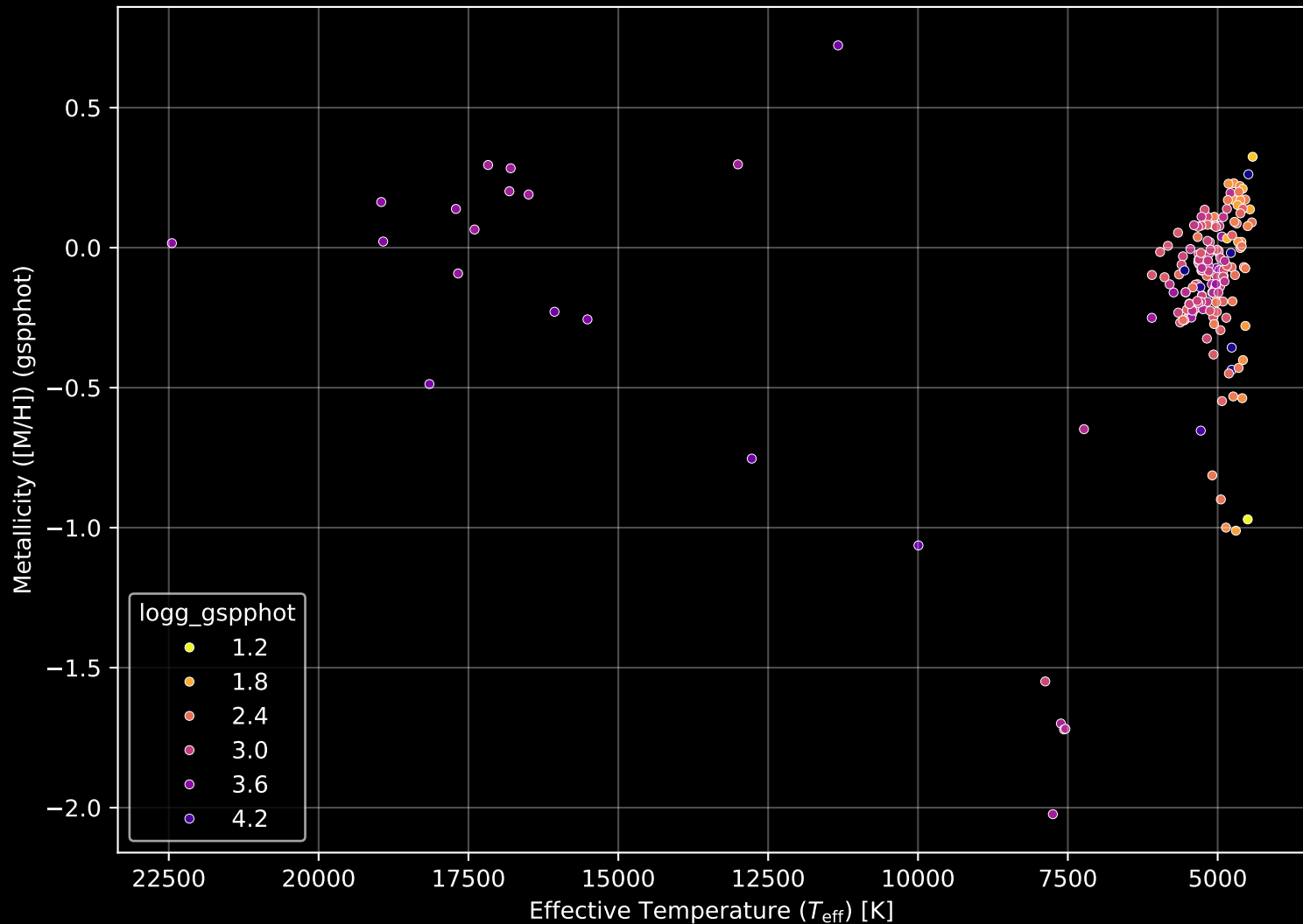
APOGEE DR17 Field: [128-04] Stellar Population Parameters (n= 182)
